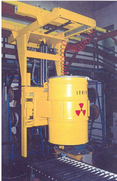
Manipulación y volteado de bidones
