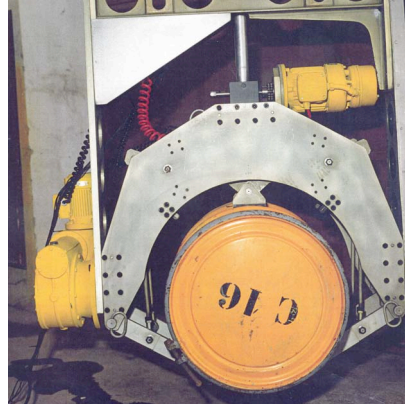
Volteado de bidones de distintos tamaños
