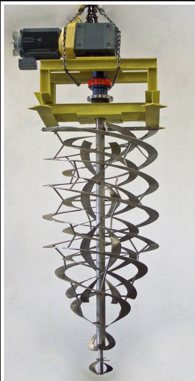
AGITADOR MEZCLADOR DE ALTAS RPM NUCLENOR - C. N. SANTA MARÍA DE GAROÑA
